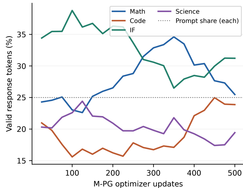
F1b Equal prompts, unequal token shares
