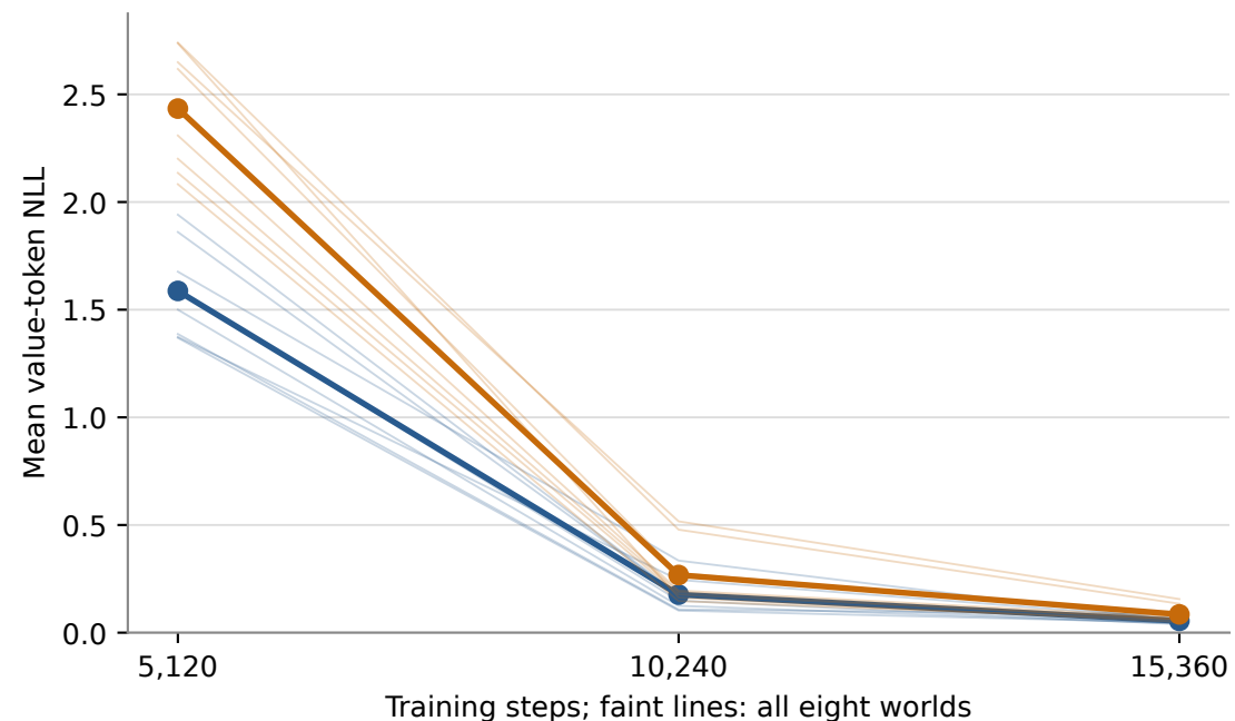
(d) Foundation-fact learning trajectories
