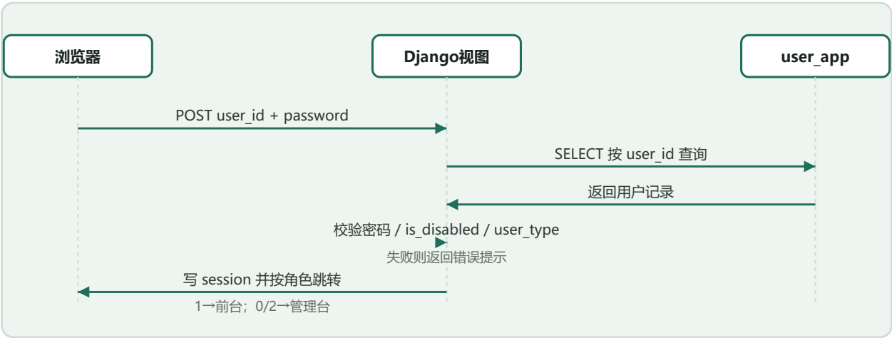
图 2 登录时序图
