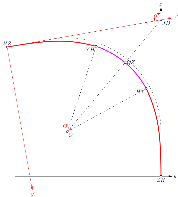
图 7.7 左偏缓和曲线的 HZ 部分坐标计算
