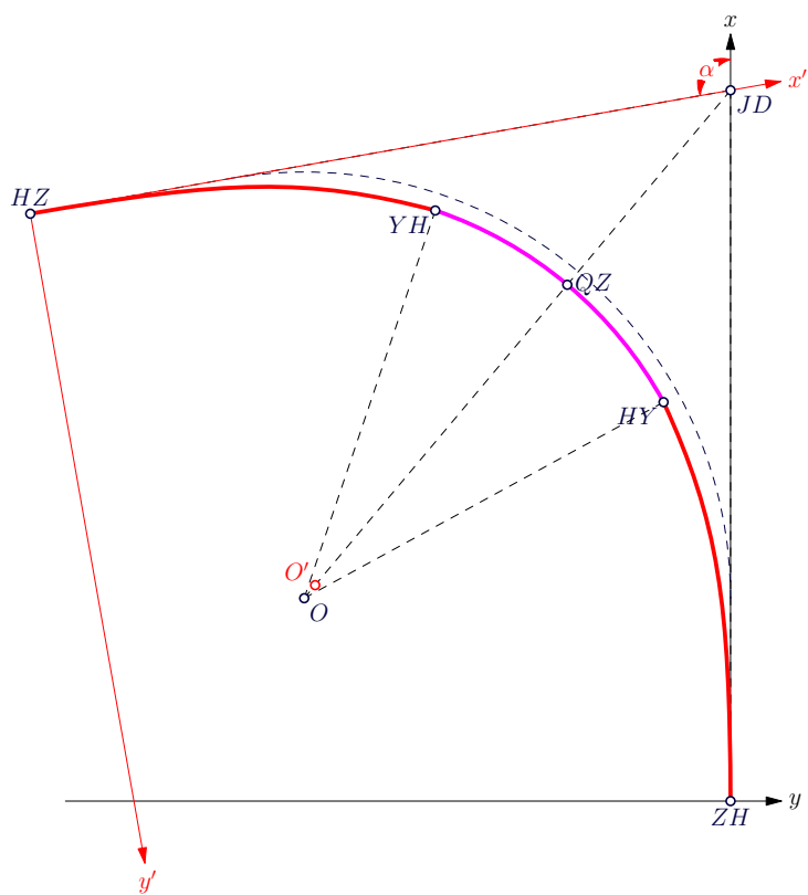
图 7.7 左偏缓和曲线的 HZ 部分坐标计算
