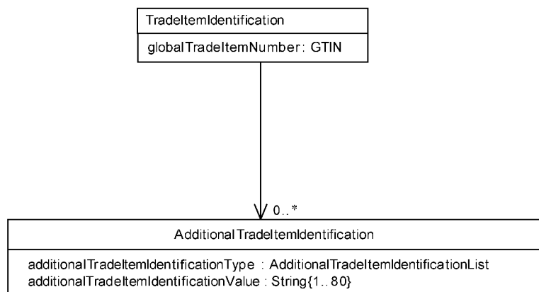
图 8 贸易项目标识类图
