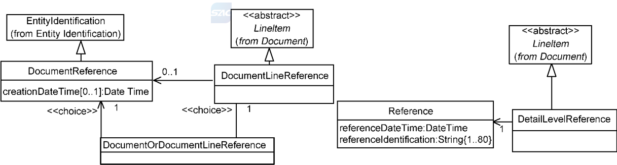
图 11 文档参考类图
