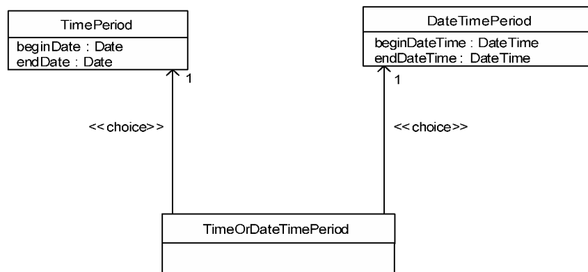
图 12 日期和时间类图
