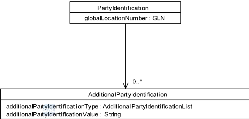
图 5 参与方标识类图
