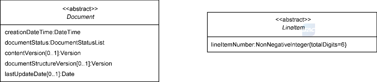
图 3 文档类图
