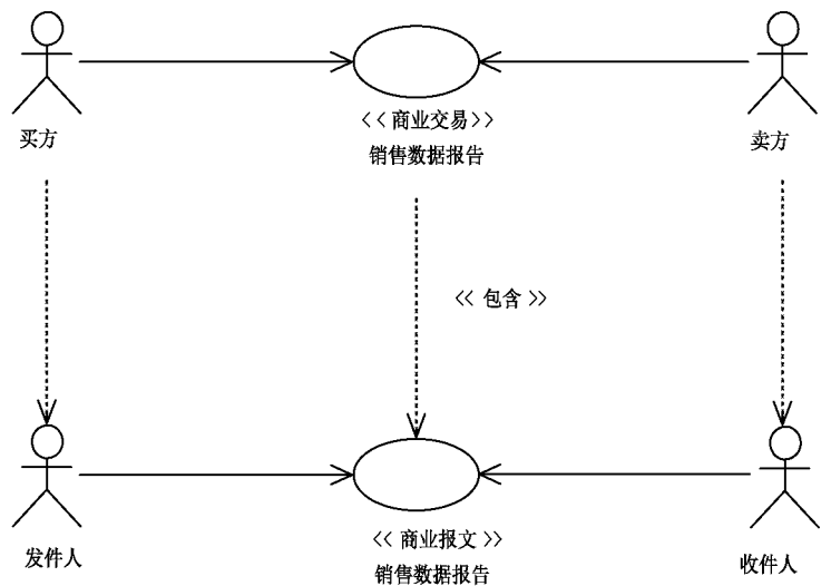
图 1 用例图
