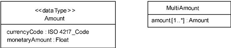
图 10 数量类图
