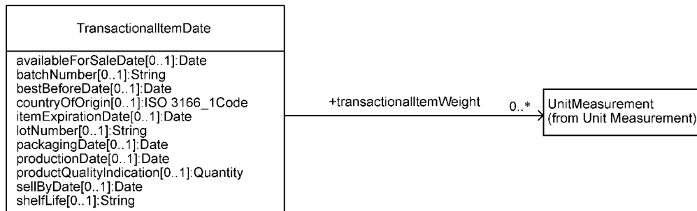
图 13 交易项目数据类图
