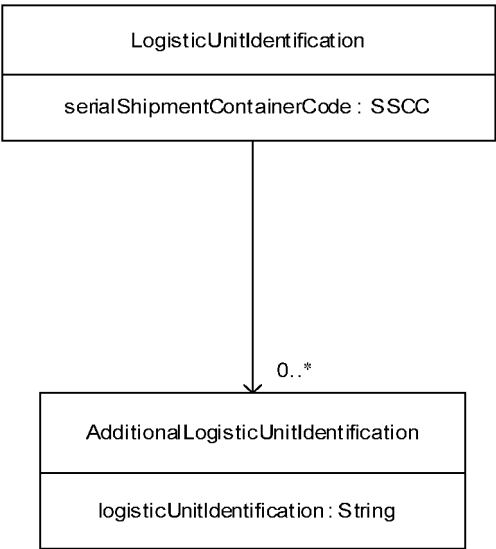
图 9 物流单元标识类图
