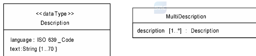
图 7 描述类图
