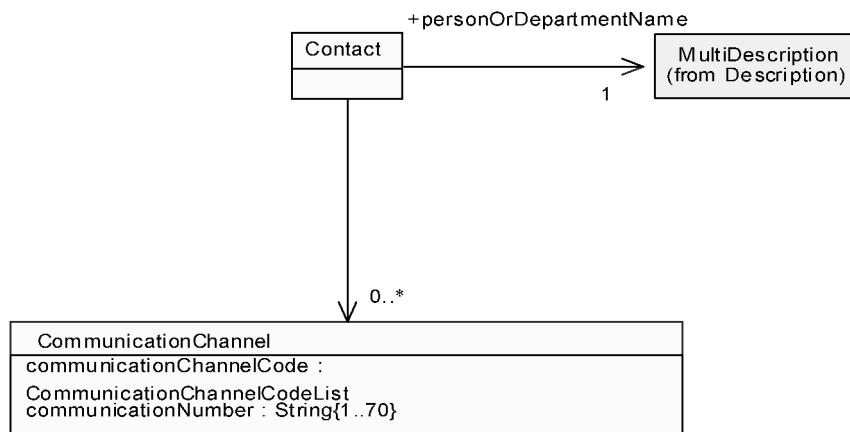
图 6 联系人类图
