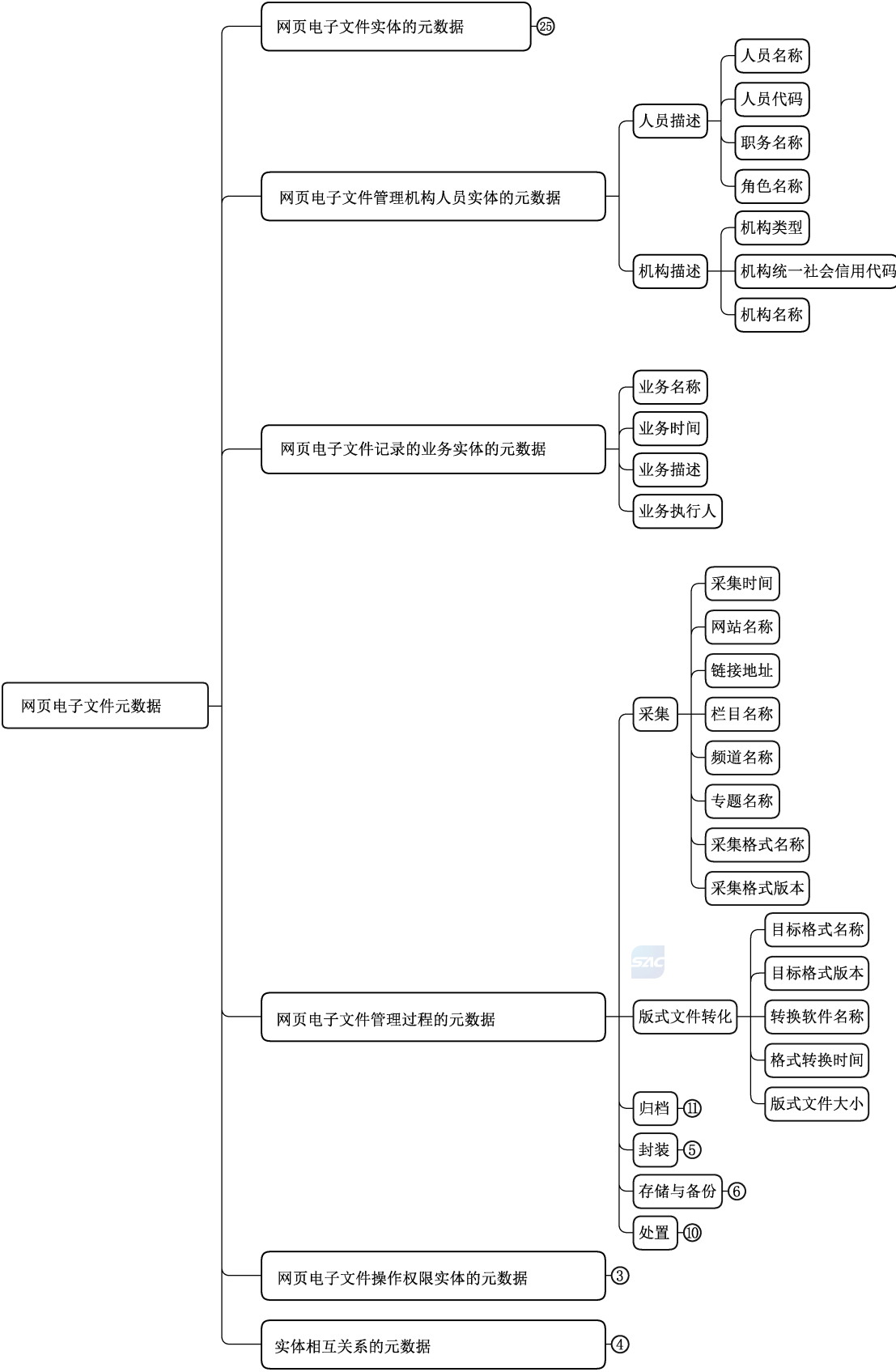
图 A.1 网页电子文件元数据的 XML Schema 结构图(续)
