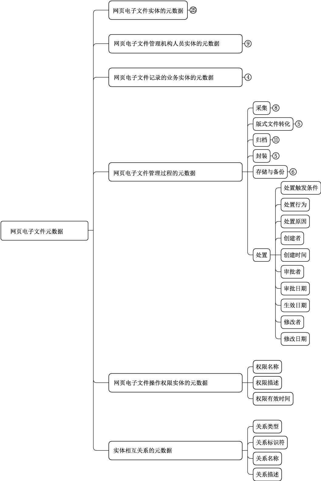
图 A.1 网页电子文件元数据的 XML Schema 结构图(续)
