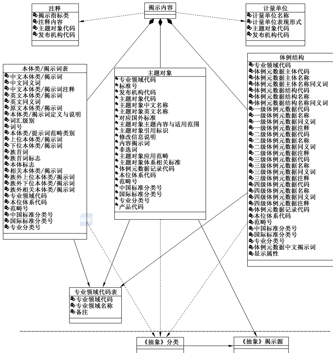
图 3 揭示核心元数据
