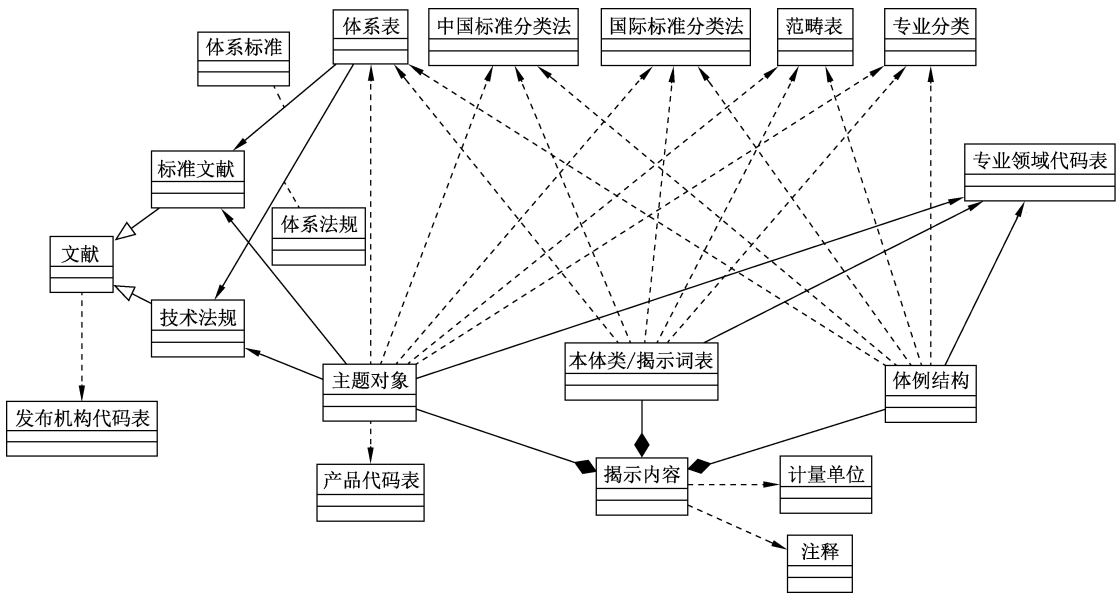
图 2 揭示元数据总图
