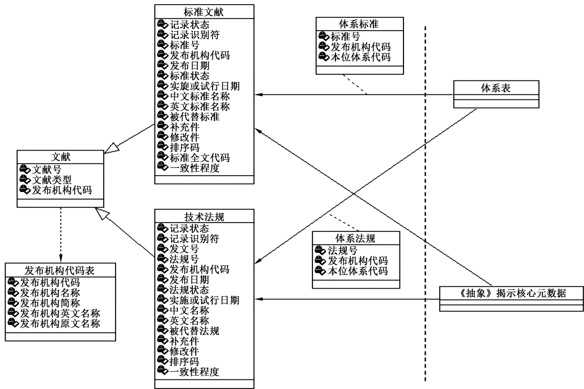
图 5 揭示源元数据
