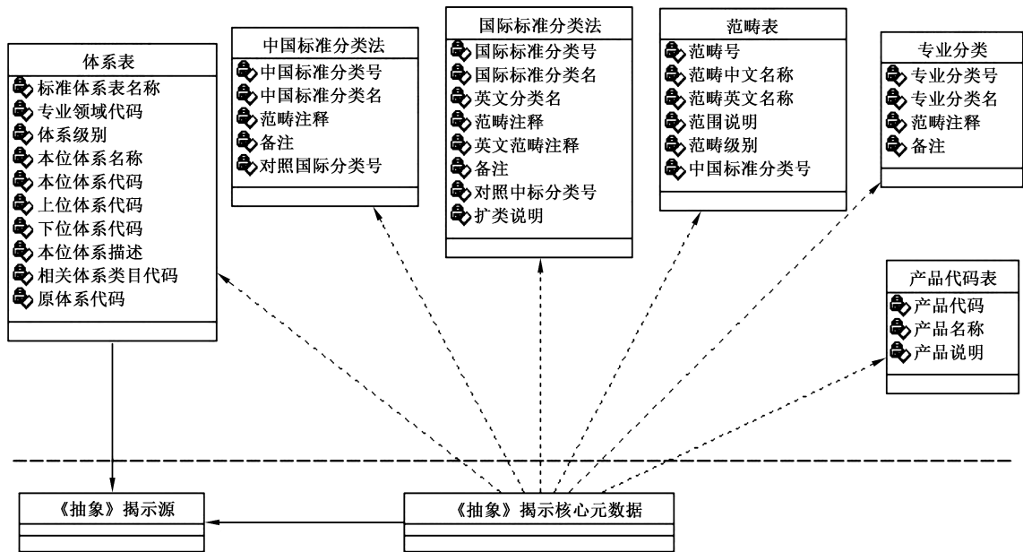
图 5 揭示源元数据
