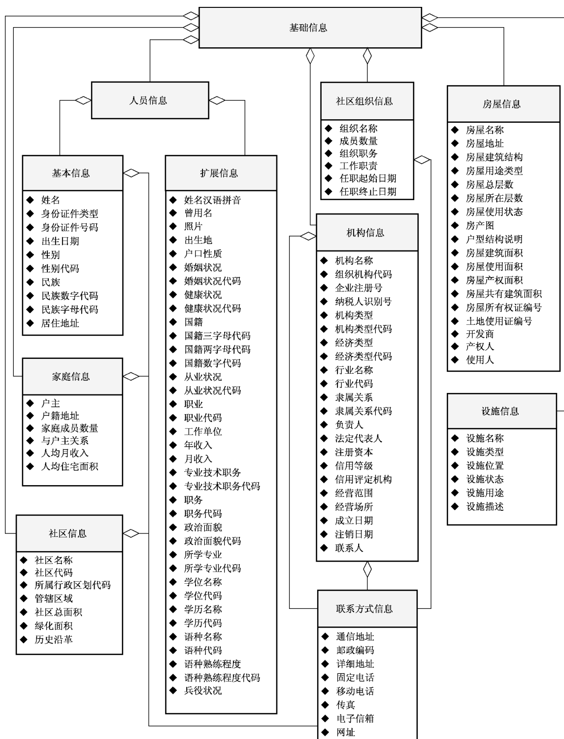
图2 社区基础数据元-基础信息-模型
