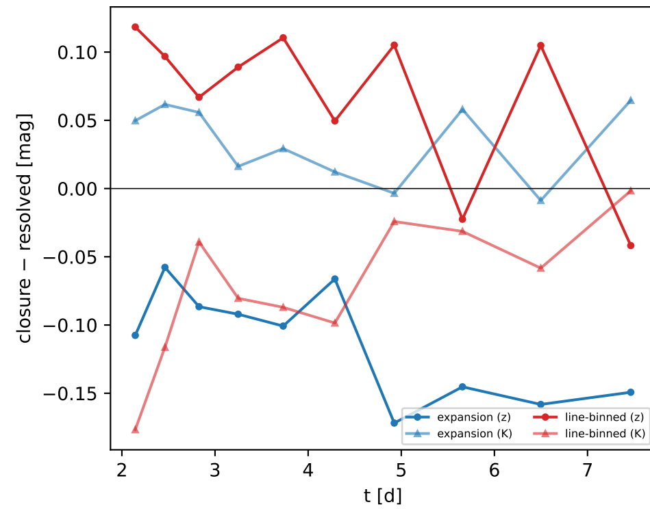
band residuals (z circles, K triangles)
