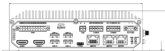
接口图
