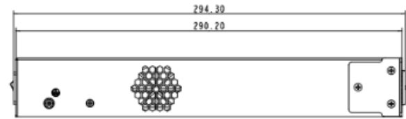
侧视图
