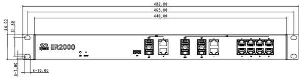
接口图
