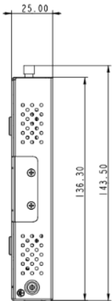
侧视图
