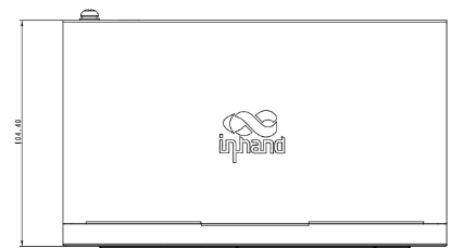
正视图
