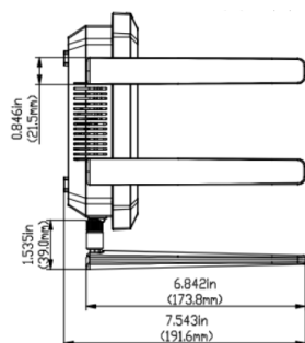
侧视图
