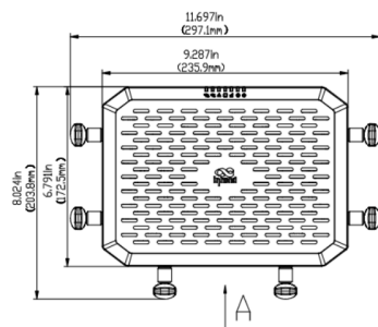
正视图
