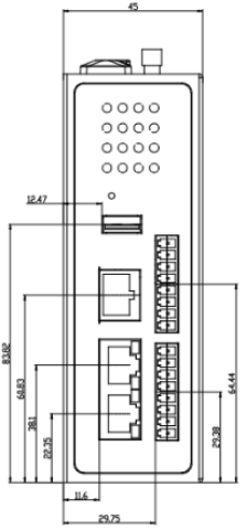
接口图
