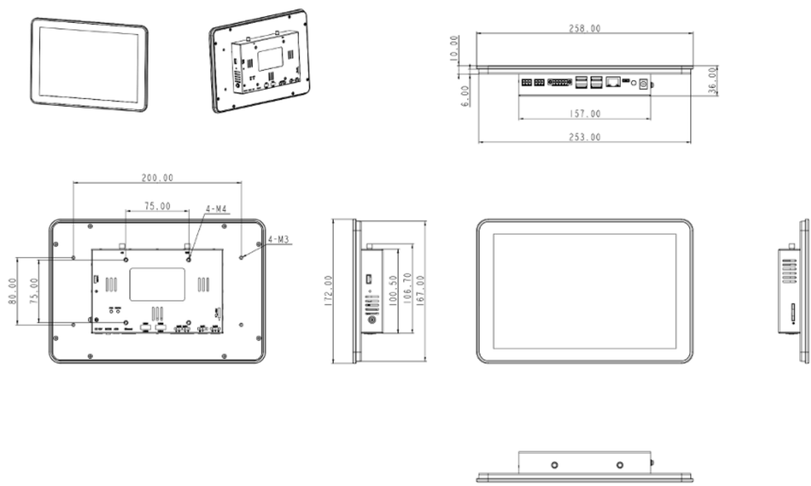
产品尺寸图
