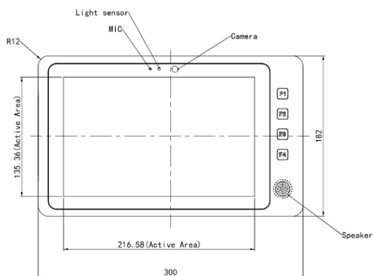
正视图
