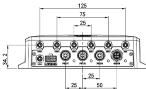
接口图
