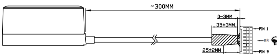
图 1.6 雷达 HY2.0 9 PIN 接口 (单位: mm)
