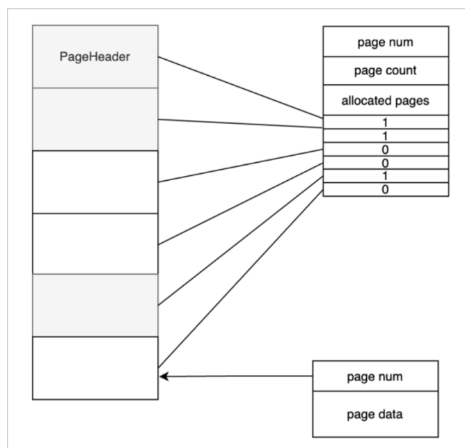
图 3: 文件结构图
