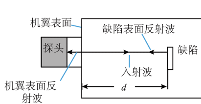
图 (a) 超声波检测原理示意图
