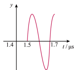
图 (c) 缺陷表面反射信号
