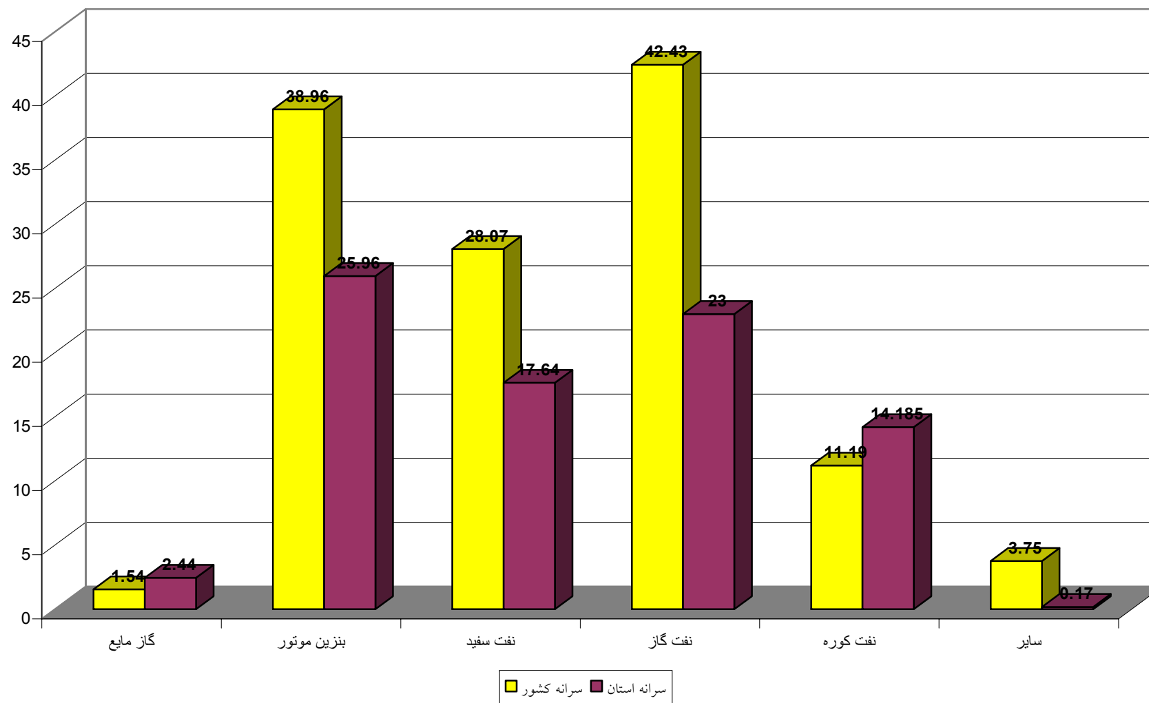
نمودار ۸. سرانه ظرفیت انبارهای نفتی استان تهران
