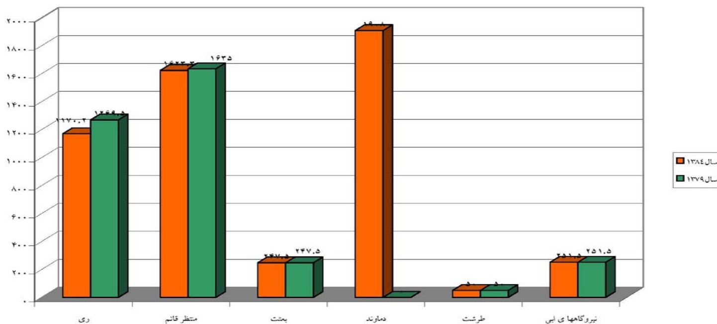
نمودار (۳۵) مقایسه میزان ظرفیت نامی نیروگاه های مختلف استان تهران در سال ۷۹ و ۸۴
