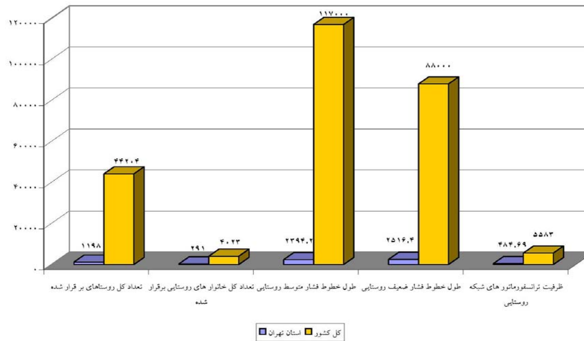
نمودار (۲۱) مقایسه شرایط برق رسانی روستاهای استان تهران و کل کشور در سال ۷۹
