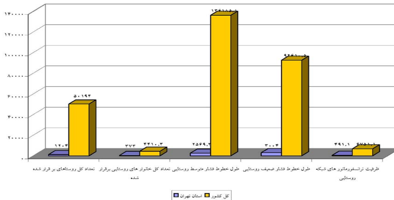
نمودار (۲۲) مقایسه شرایط برق رسانی روستاهای استان تهران و کل کشور در سال ۸۴
