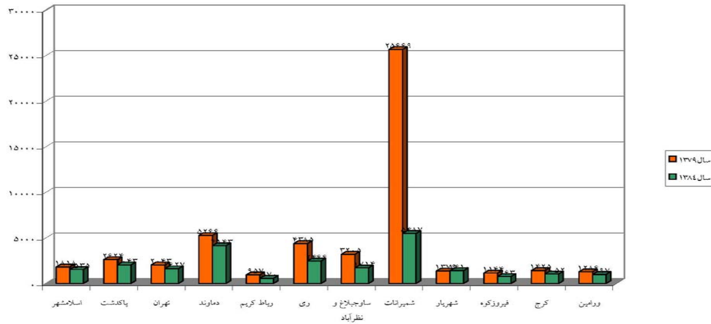
نمودار (۵۰) مقایسه سرانه فروش برق شهرستان های مختلف استان تهران در سالهای ۱۳۷۹ و ۱۳۸۴
