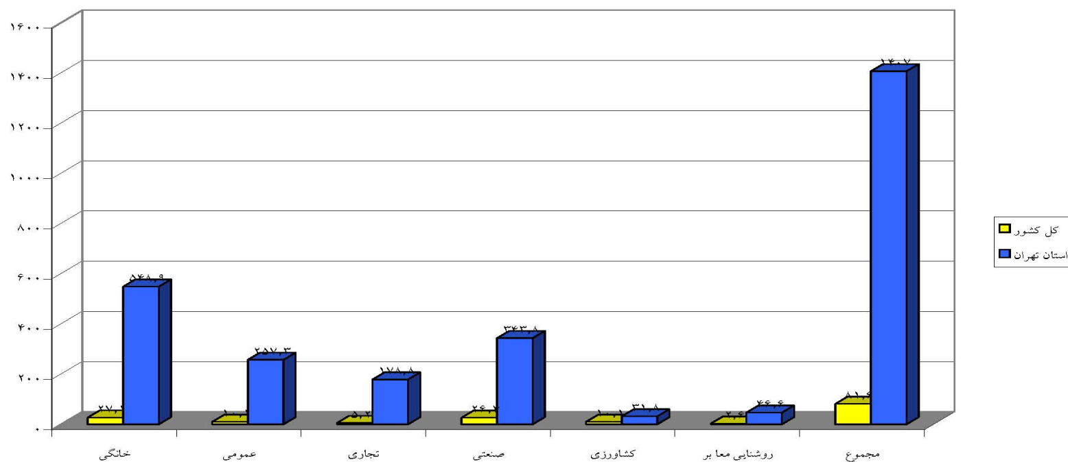
نمودار (۳۲) مقایسه شاخص فروش برق بر واحد سطح در استان تهران و کل کشور در سال ۱۳۸۴
