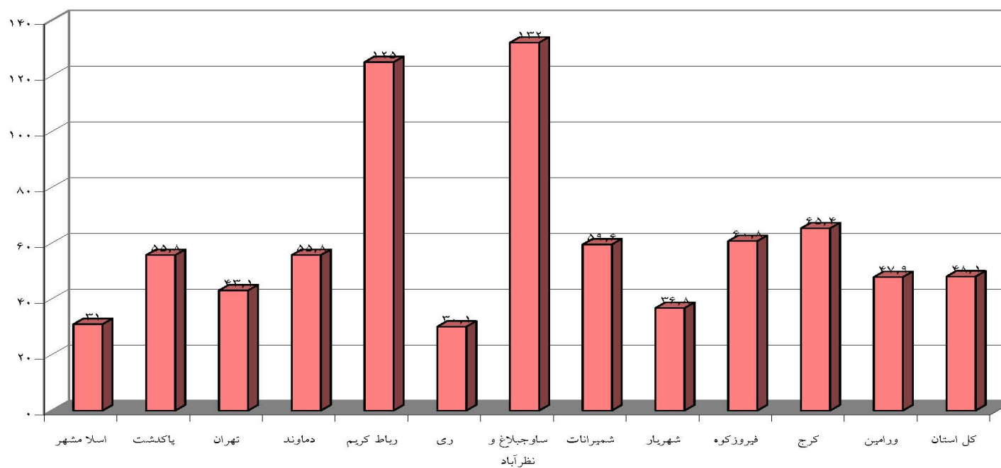
نمودار (۵۷) مقایسه درصد رشد شاخص مصرف انرژی برق بر واحد سطح در شهرستان های مختلف استان در سال ۸۴ نسبت به ۷۹
