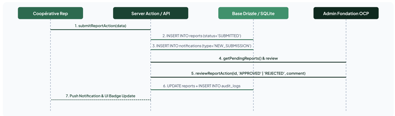
Diagramme de Séquence : Circuit de Validation des Rapports
