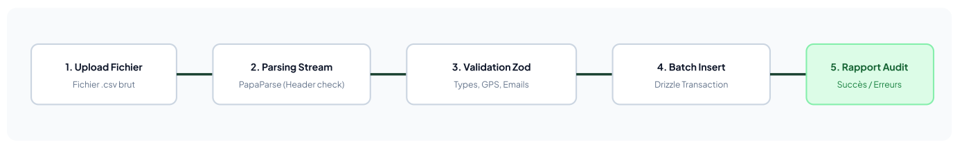
Pipeline ETL de Traitement des Fichiers CSV
