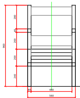
ALÇAT
