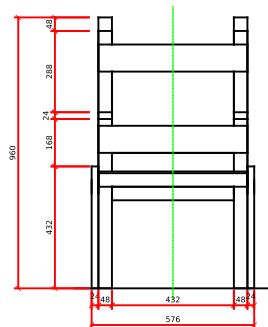
ALÇAT
