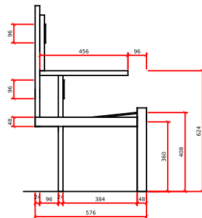
PERFIL ESQUERRE
