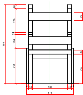
ALÇAT
