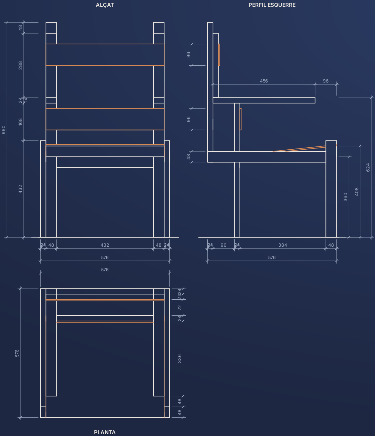
Escala 1:10 · cotes en mm · sistema europeu
