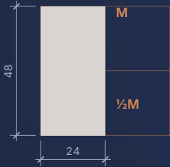
Secció del llistó, E 1:2
