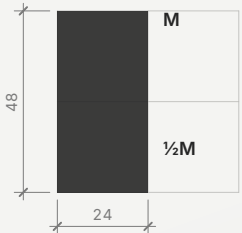
Secció del llistó, E 1:2
