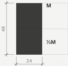
Secció del llistó, E 1:2
