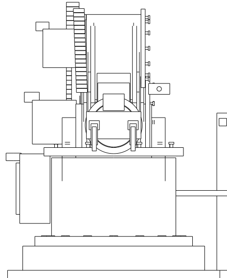
右视图 / RIGHT VIEW
