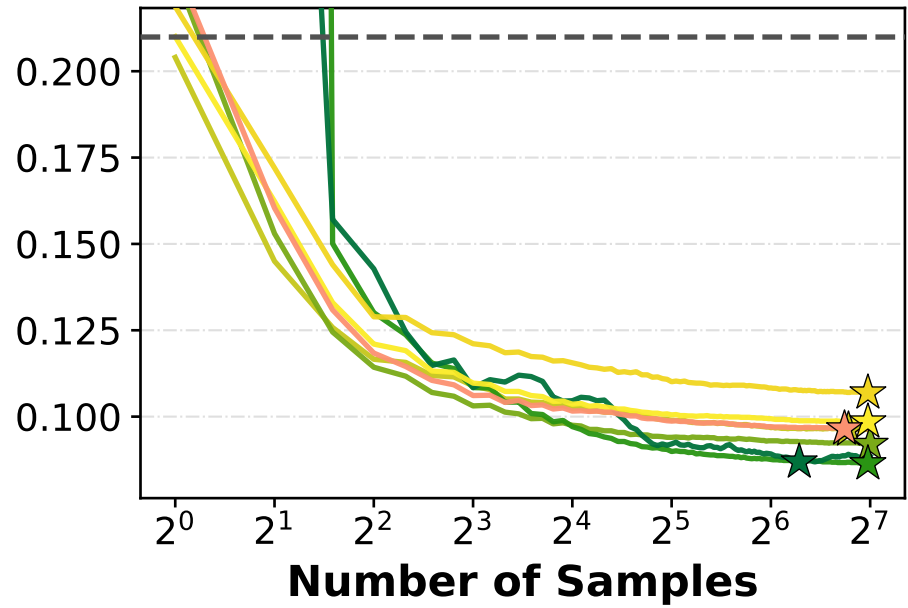
Moirai
