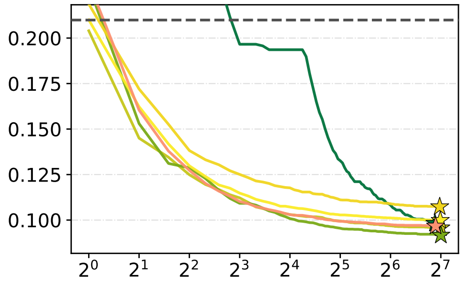
Moirai
