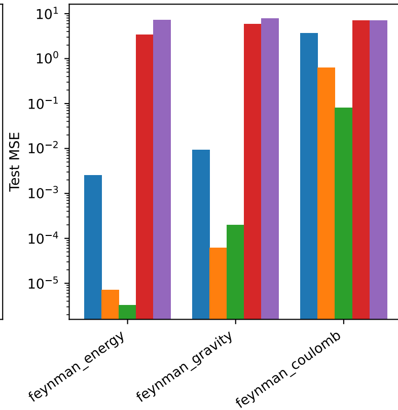
Test MSE
