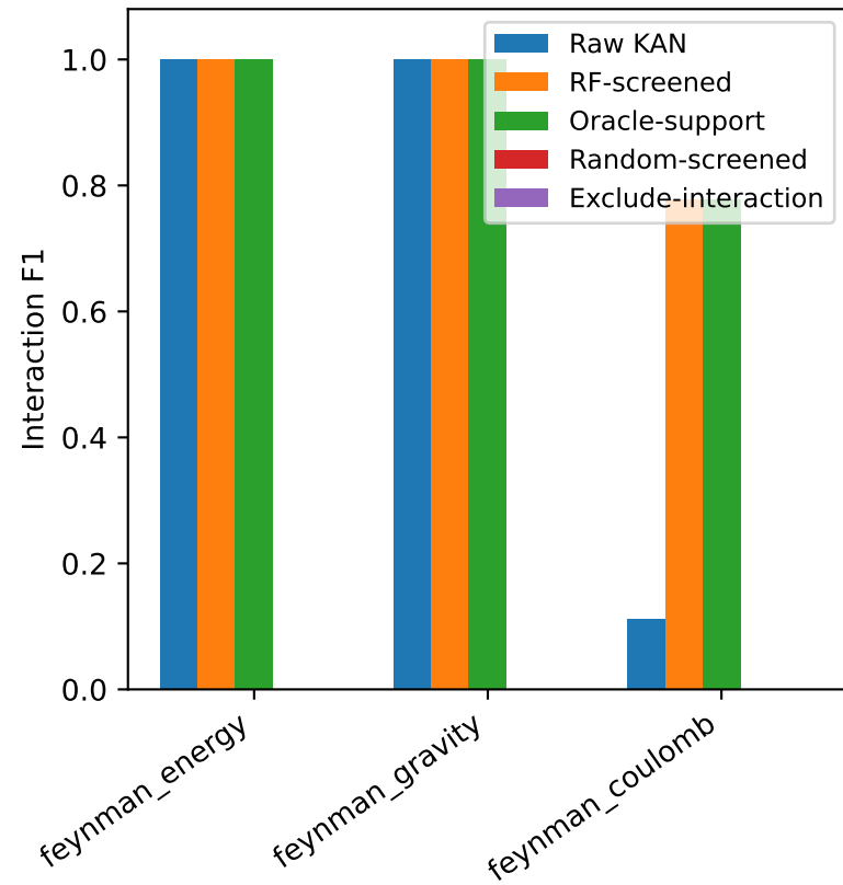
Interaction F1
