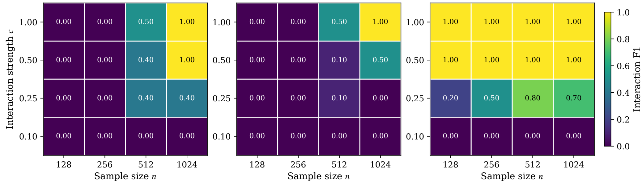
Raw KAN
