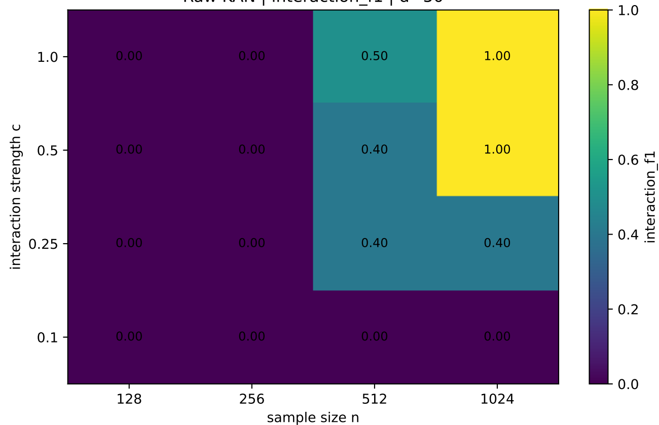
Raw KAN | interaction_f1 | d=50
