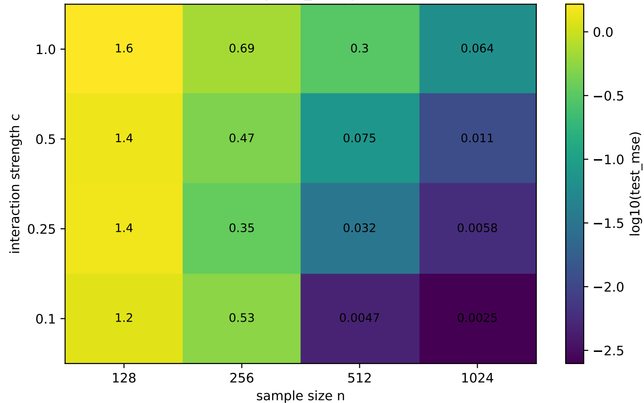
Raw KAN | test_mse | d=100
