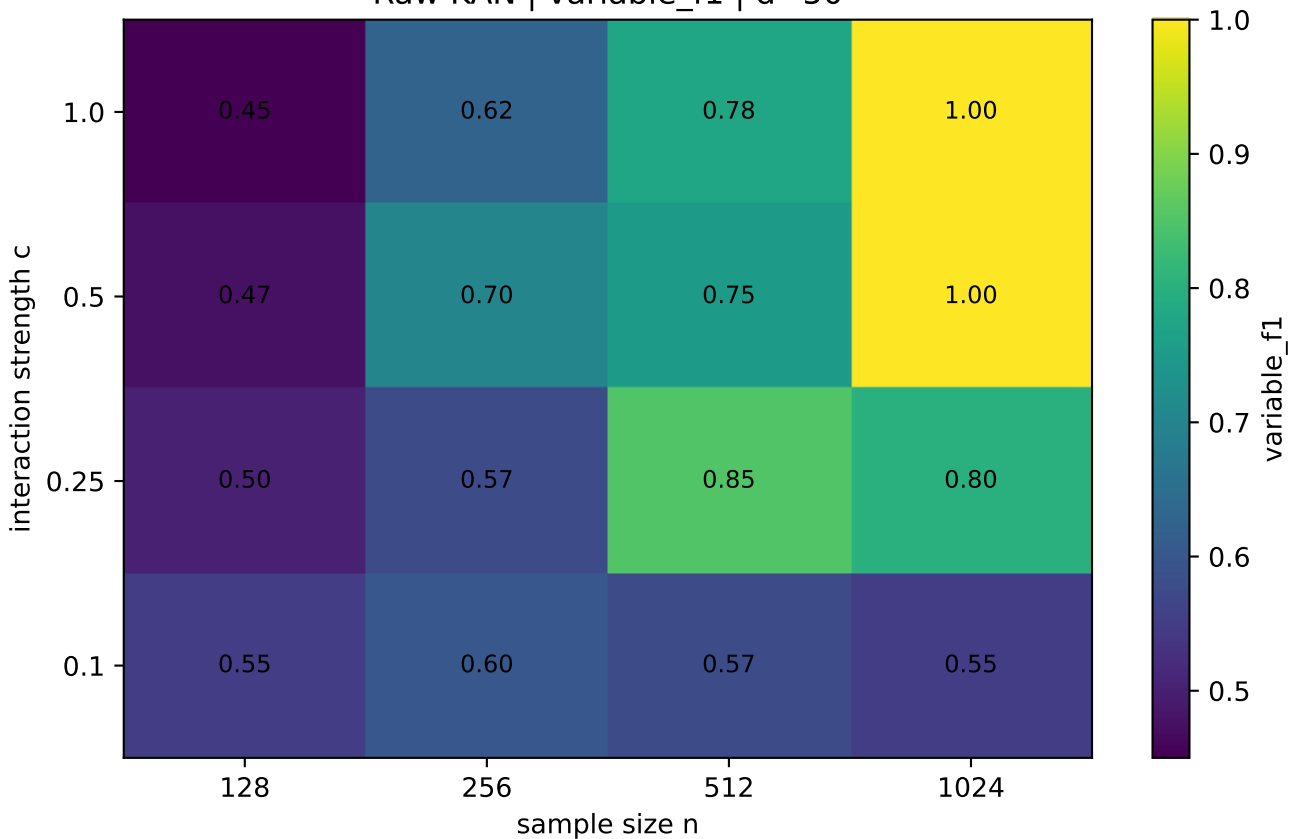
Raw KAN | variable_f1 | d=50
