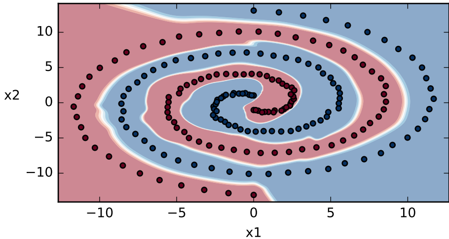
MLP
