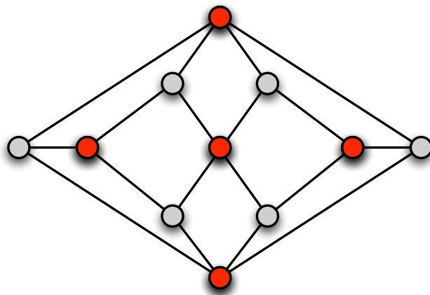
Slika 3.1: Herschelov graf, vektorska grafika.
