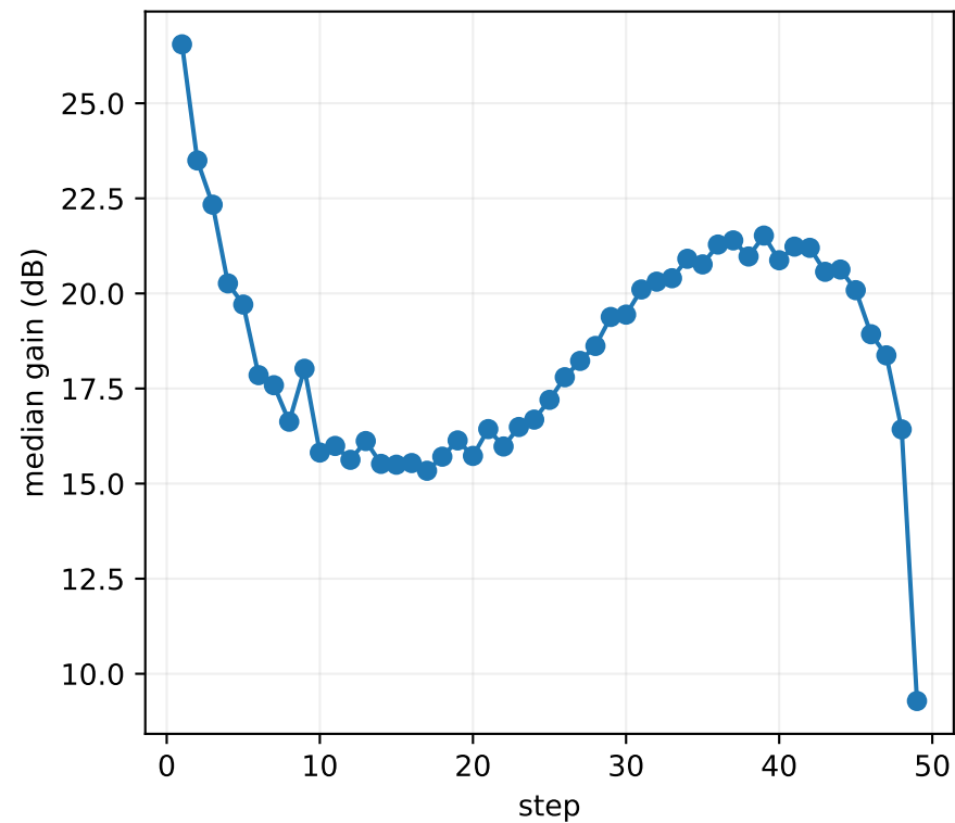
DIT
