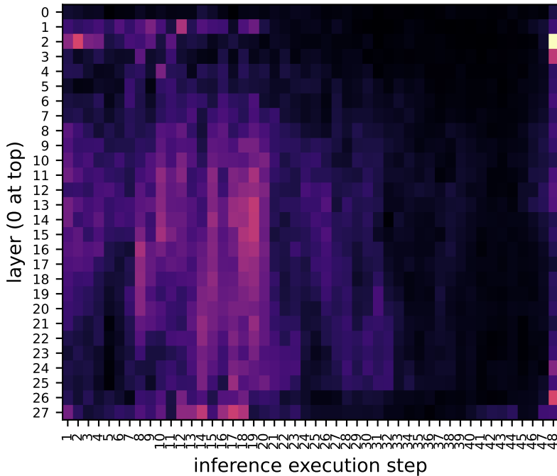
dit.mlp
