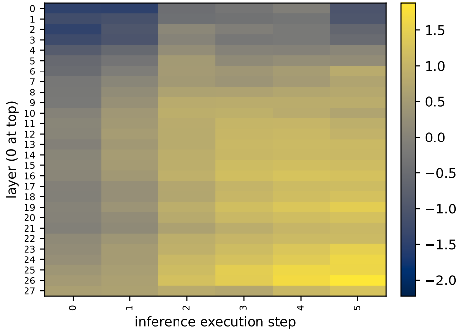
dit.msa
