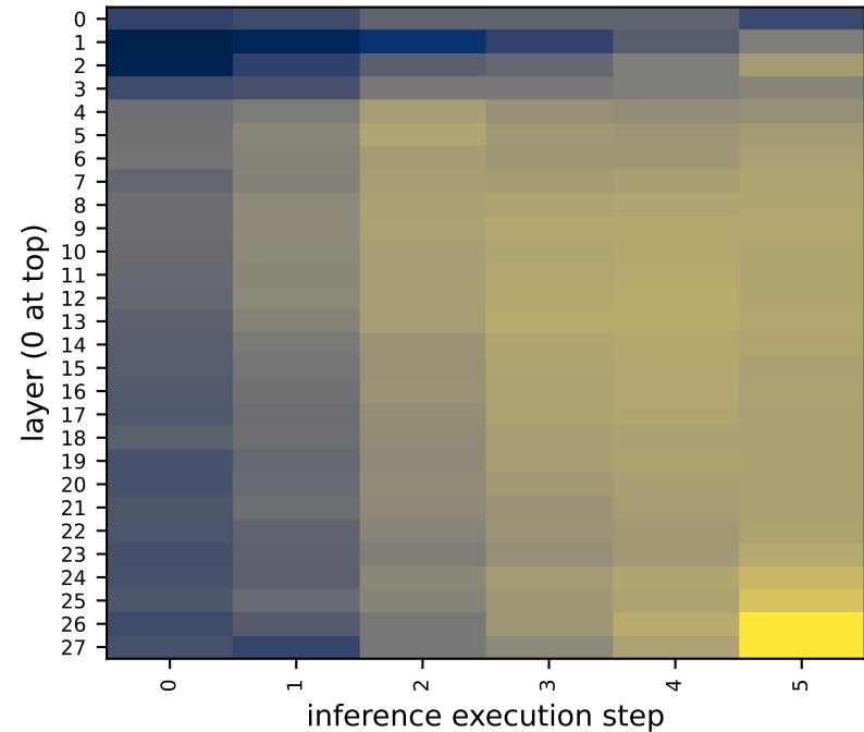
dit.mlp
