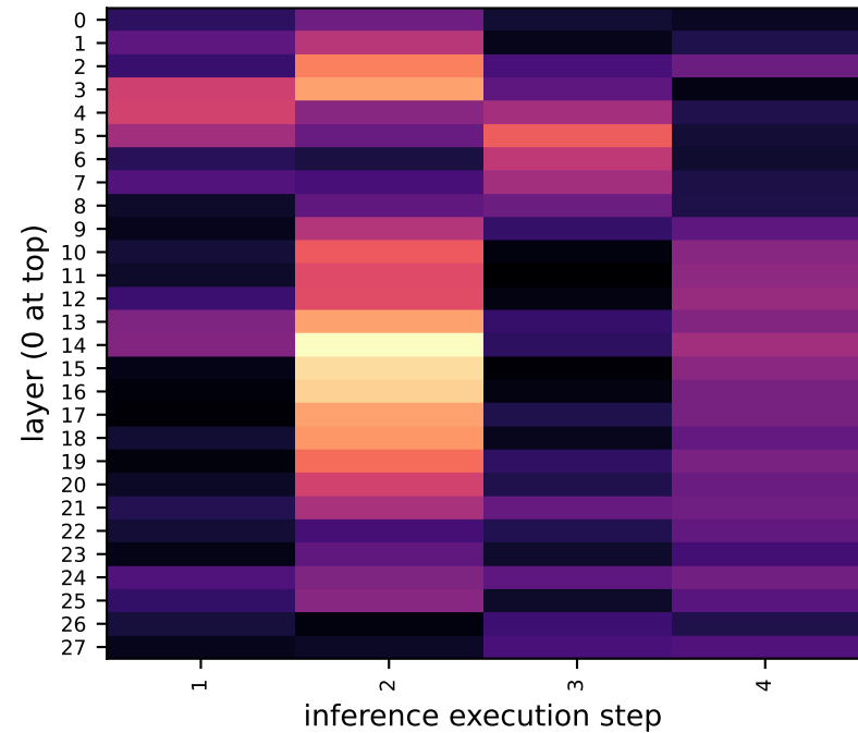
dit.mlp
