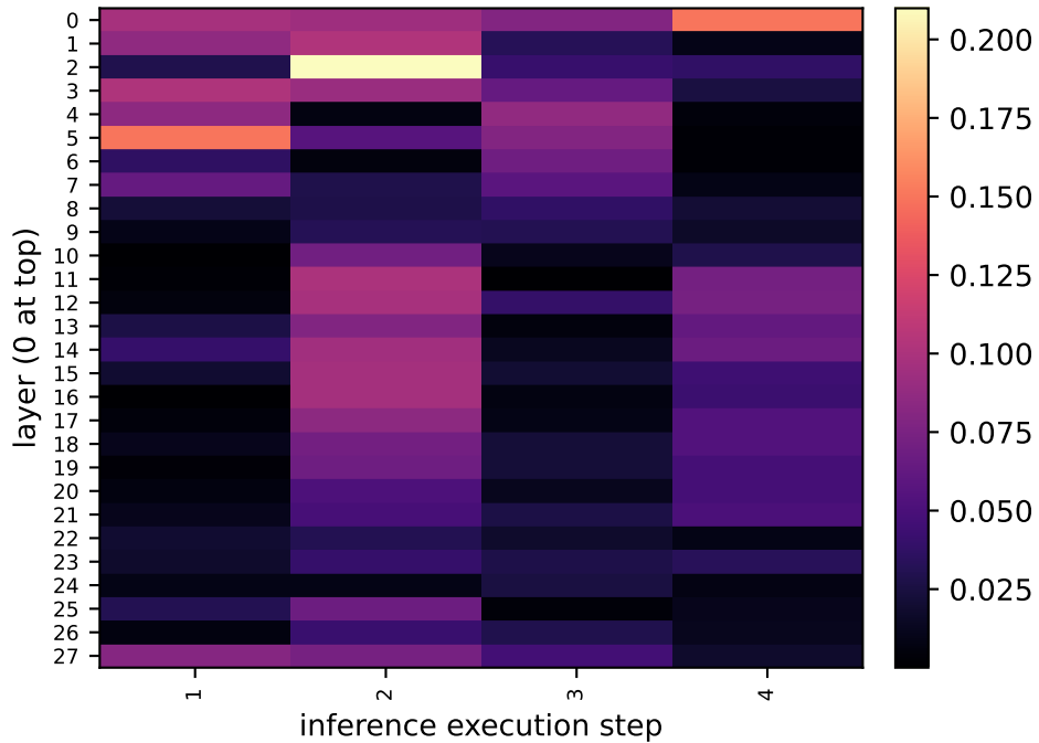
dit.msa
