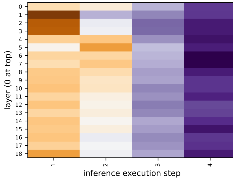
single.attn
