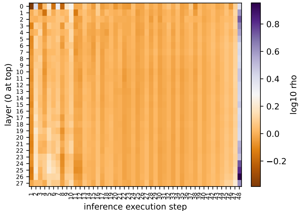
dit.msa
