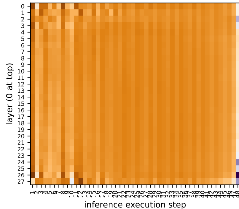
dit.mlp
