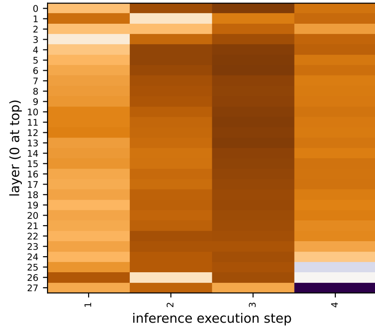
dit.mlp
