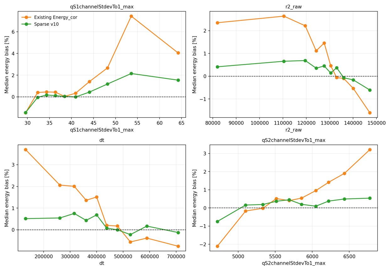
图 9 前四个关键变量分箱后，已有三次式与 v10 的能量偏差趋势。绿色曲线更接近零表示相应条件依赖被减弱。
