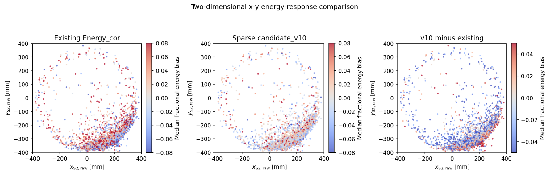
图 12 已有三次式、v10 与二者差异的 x - y 逐事件偏差图。颜色表示相对 2,614.5 keV 的逐事件偏差，不是事件密度。
