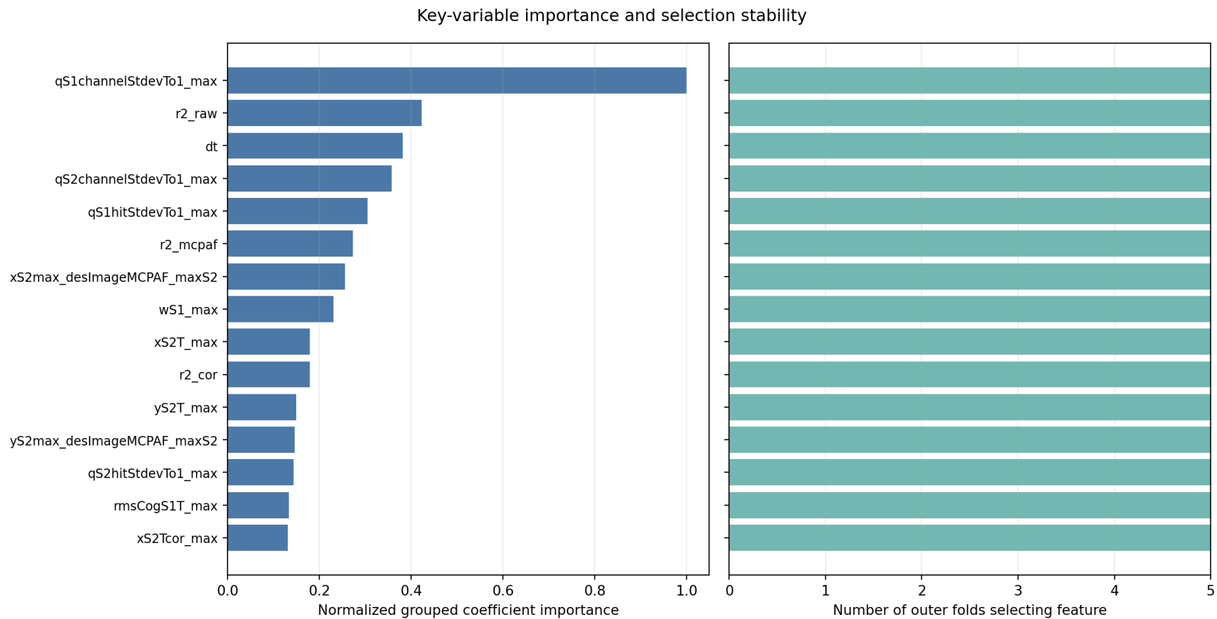
图 8 关键变量的重要性 with 五个外层训练池中的入选稳定性。重要性用于排序，不表示唯一因果贡献。
