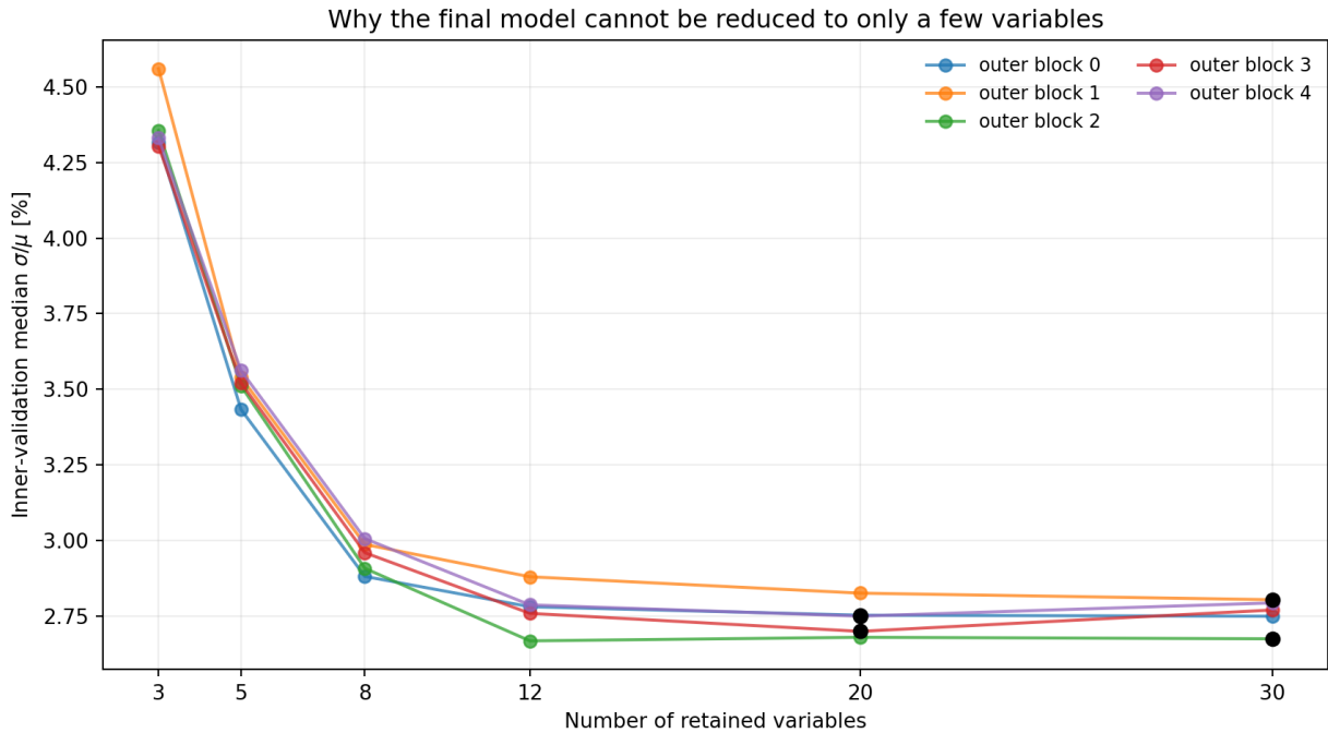
图 7 不同变量数量在五个外层训练池内部验证中的表现。黑点为各外层流程选择的 k 。
