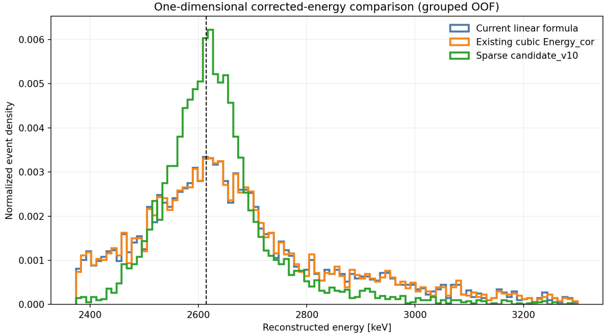
图 10 三种重建方法在同一批合并 OOF 事件上的归一化一维能谱。v10 的中心峰更高、更窄，但仍保留可见尾部。
