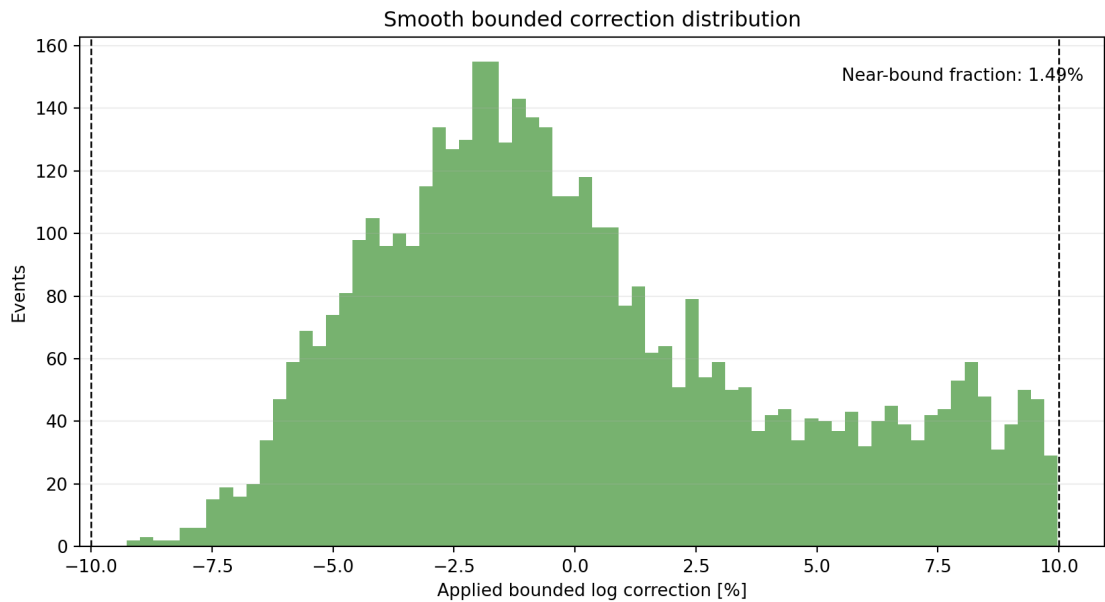
图 13 v10 的单事件对数修正分布。虚线为平滑上限±0.10。
