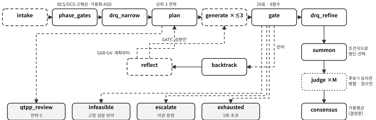
그림 5. 후보 탐색 그래프. backtrack은 반려 판정을 전이표에 대조해 복귀 지점(GATE: 같은 전략으로 성분만 교체, G6R: 공정 경로부터, G4: 전략 선택부터)과 제약을 정한다. 하단은 종결 노드이다.
