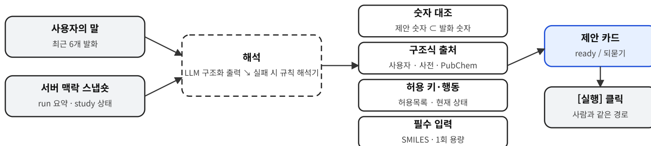
그림 2. 입력 에이전트의 처리 경로. 해석(LLM, 실패 시 규칙 해석기) 이후의 가드레일은 모두 코드로 구현되어 있다.
