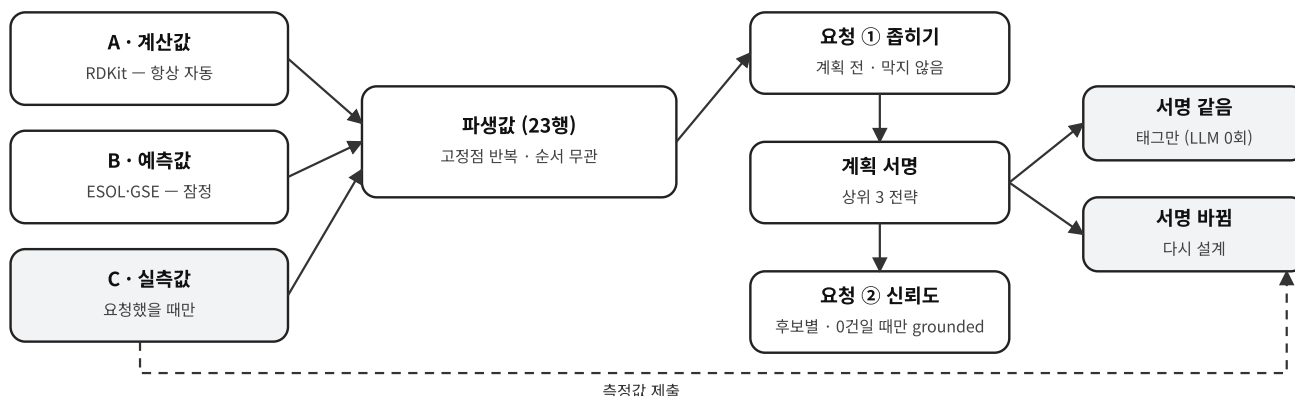
그림 3. 값의 세 계층과 비차단 실험 요청. 측정값이 입력되면 그래프를 다시 실행하지 않고 결정론 계층만 재계산하며, 계획 서명이 같으면 신뢰도 태그만 갱신한다.
