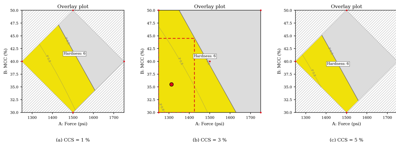
그림 8-2. CBD 13단계 Overlay plot(CCS (a) 1, (b) 3, (c) 5 % 단면). 기준은 게이트를 통과한 경도의 평균 예측(4~6 kgf)이다. 빨간 점선은 control space, 큰 빨간 점은 최적 처방, 회색 점선은 보조 확률(0.5, 0.8)을 나타내며, 형식은 논문 Figure 2와 같다.
