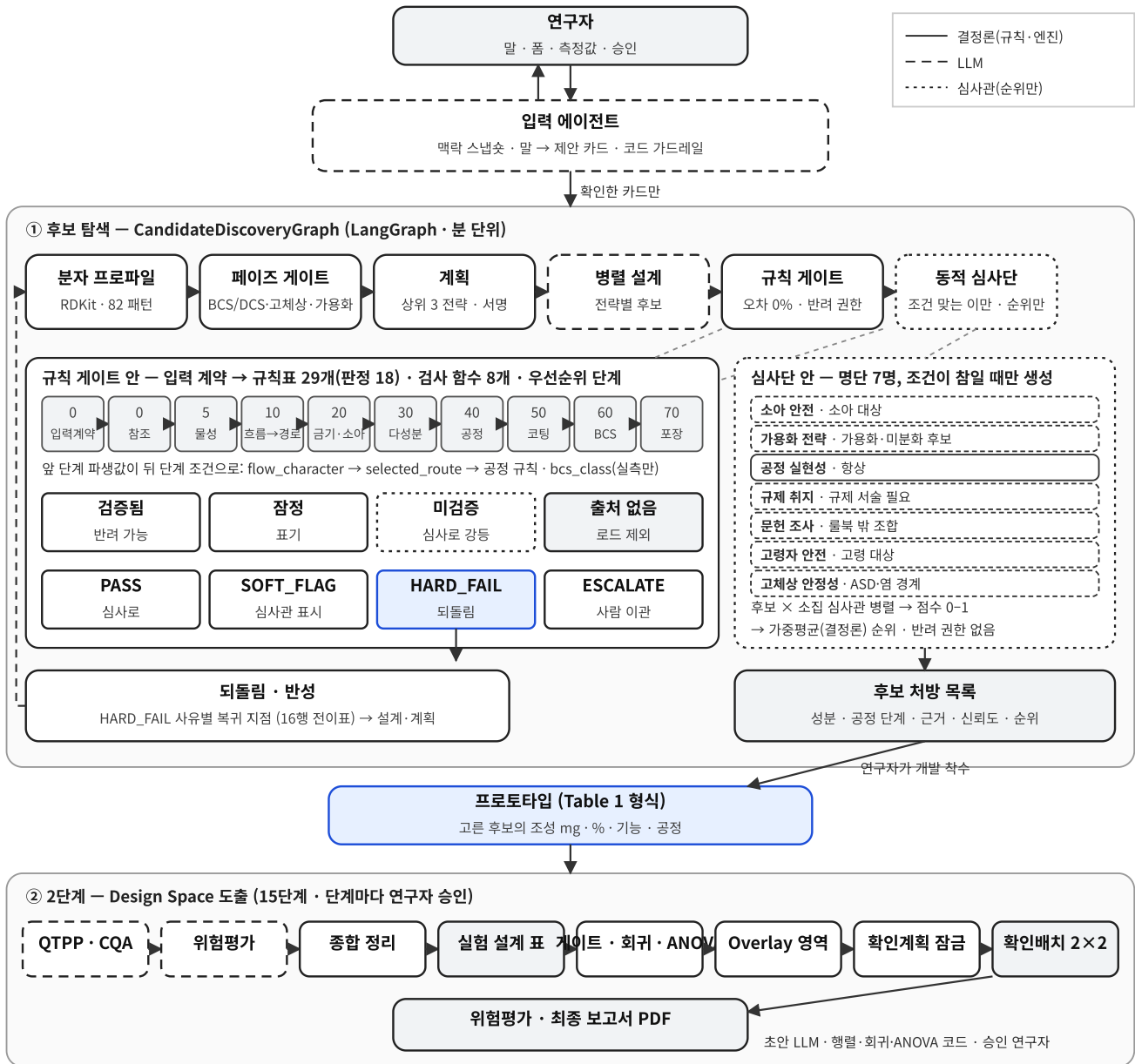
그림 1. 전체 구조. 연구자와 두 그래프 사이에 입력 에이전트가 있으며, 두 단계는 내부 상태를 공유하지 않고 연구자가 선택한 후보의 처방(프로토타입) 하나로만 연결된다. ① 안의 두 확대 상자는 규칙 게이트(우선순위 단계, 근거 상태별 권한, 판정별 경로; 그림 4)와 동적 심사단(명단 7명과 소집 조건, 순위만 매기는 합의; 그림 6)의 내부 구조이다. 선 모양은 담당 주체를 나타낸다(실선: 결정론 규칙·엔진, 파선: LLM, 점선: 순위만 매기는 심사관).
