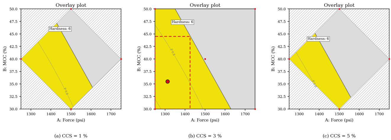
그림 10. CBD 13단계 Overlay plot(CCS (a) 1, (b) 3, (c) 5 % 단면). 기준은 게이트를 통과한 경도의 평균 예측(4~6 kgf)이다. 빨간 점선은 control space, 큰 빨간 점은 최적 처방, 회색 점선은 보조 확률(0.5, 0.8)을 나타내며, 형식은 논문 Figure 2와 같다.
